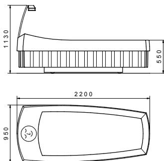
Maße AquaThermoJet
