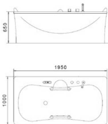
Maße Vis à Vis 1000
