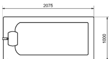
Maße AquaThermojet
