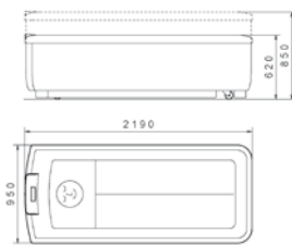
Maße Lady-Spa Standard Verkleidung
